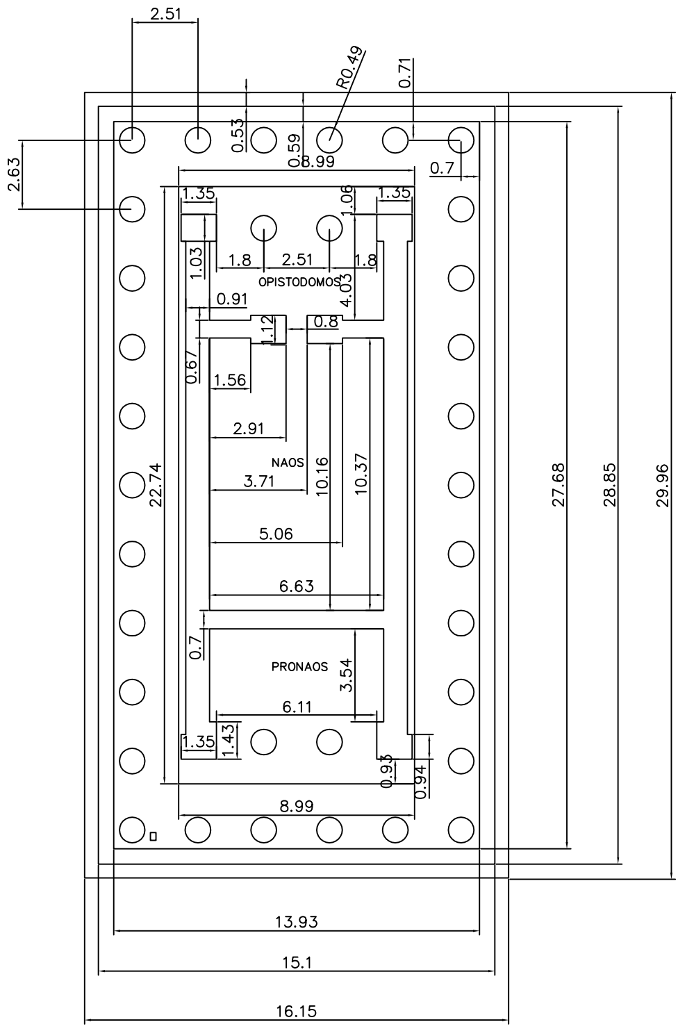
Esquema de templo dórico, hexástilo y períptero
